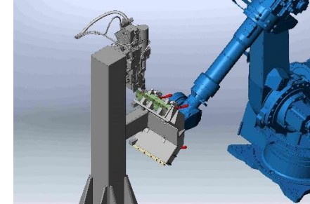
Roller hemming
